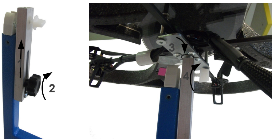
Fig. 110: Fixation de la croix centrale en position "Orienter"
