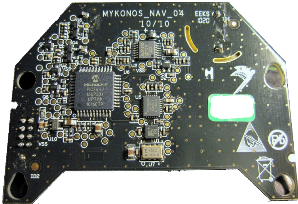
Fig. 127: face avant carte de navigation
